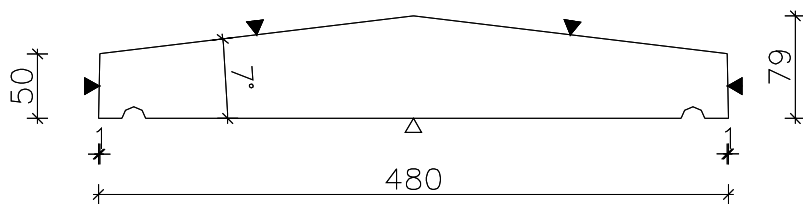
Doorsnede
