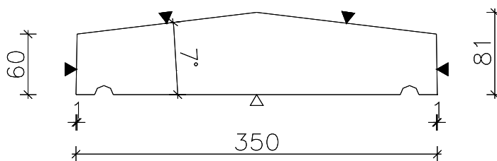
Doorsnede
