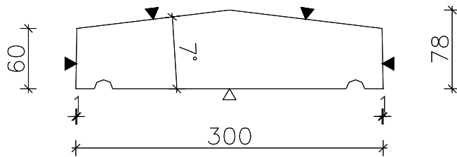
Doorsnede
