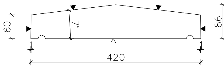
Doorsnede
