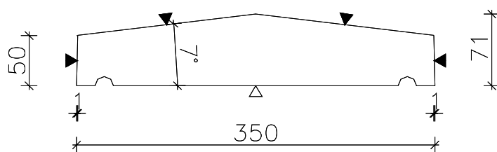
Doorsnede
