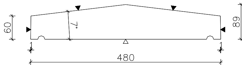
Doorsnede
