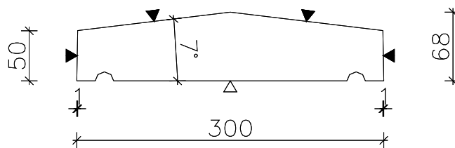
Doorsnede
